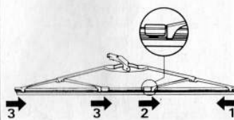
Het losmaken van het rubberprofiel voor de ruitwissers
