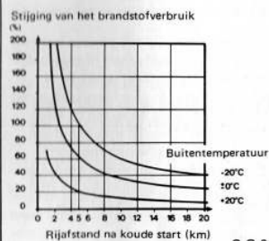
S G 012 Stijging van het brandstofverbruik bij koude start vergeleken met opgewarmde auto bij verschillende temperaturen.
