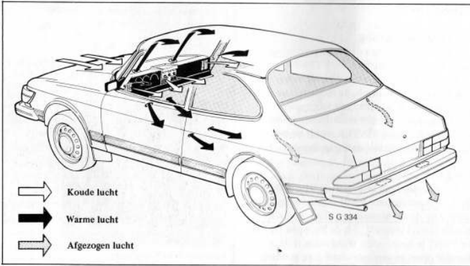
Samengestelde luchtstroom door het interieur.
