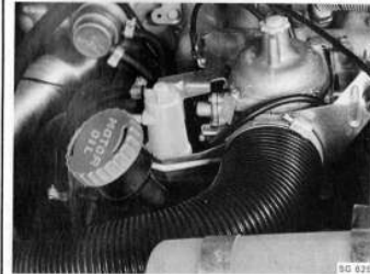
Vuldop motorolie met oliepeilstok
