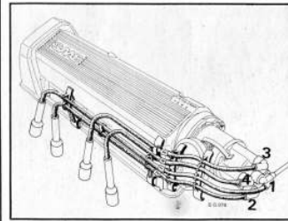
Posities van de bougiekabels
