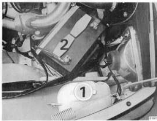
Plaatsing van de accu 1. Sproetervloeistofreservoir. 2. Accu
