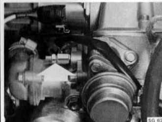
Ontluftingsnippel
