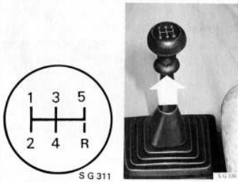
S G 311 Schakelstanden en versnellingshandel
