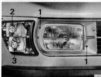
Afstelschroeven en lampen 1. Afstelschroeven, koplamp. 2. Gloeilamp, richtingaanwijzer. 3. Gloeilamp, parkeerlichten.
