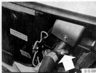
Ontluftingsnippel
