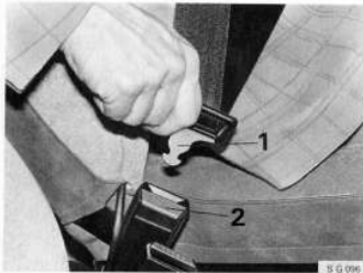
Veiligheidsgordel, voorstoel 1. Gesp. 2. Ontgrendelingsdrukknop.
