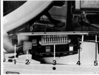
Zekeringen
