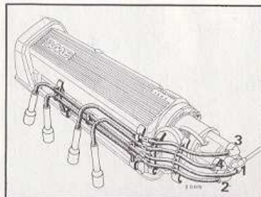
Posities van de bougiekabels
