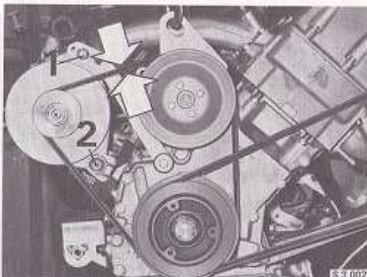
Controle spanning van de dynamoriem
