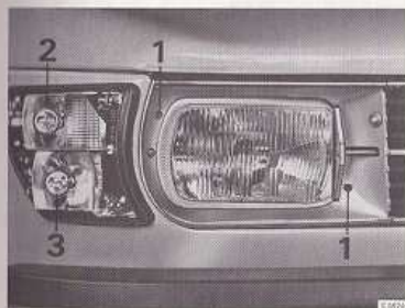
Afstelschroeven en lampen 1. Afstelschroeven, koplamp. 2. Gloeilamp, richtingaanwijzer. 3. Gloeilamp, parkeerlichten.
