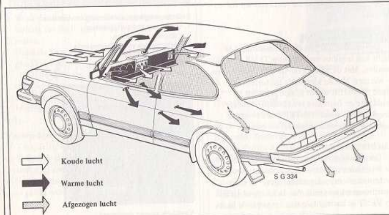
Samengestelde luchtstroom door het interieur.
