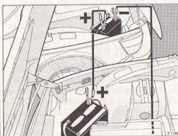
Het starten met behulp van een extra accu
