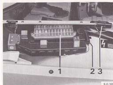
Zekeringen
