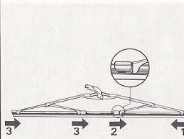
Het losmaken van het rubberprofiel voor de ruitwissers
